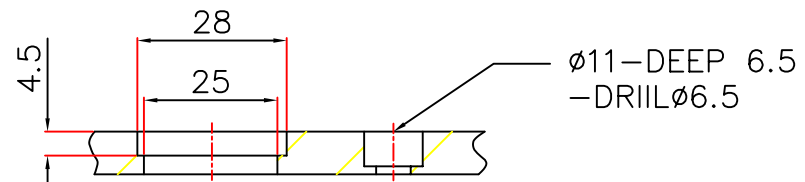
A-A 剖面
